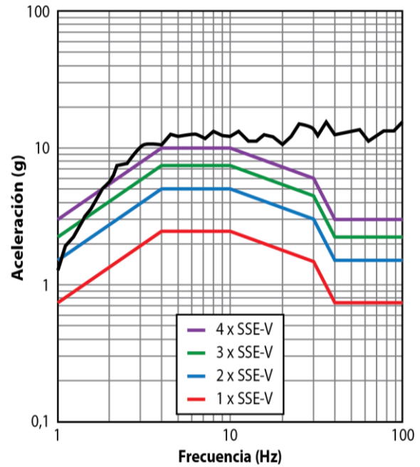
ESPECTRO DE RESPUESTA DE ENSAYO (5%) - VERTICAL
